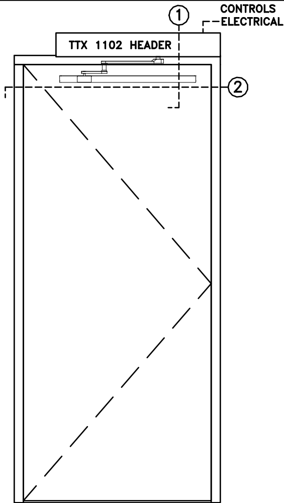
ELEVATION
