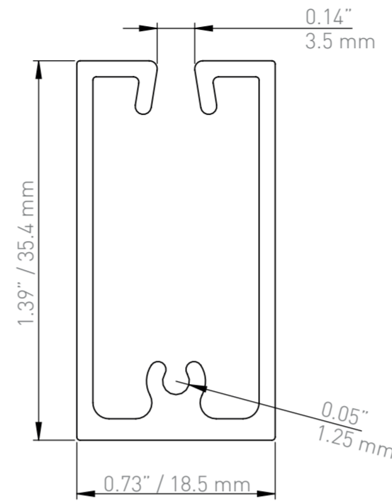
Neolux Neox Bottomrail 0-159-AL-0006X
