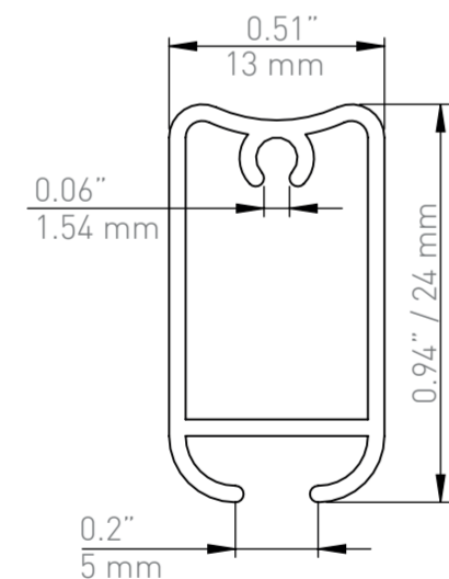
Neolux Bottomrail II 0-159-AL-0004X
