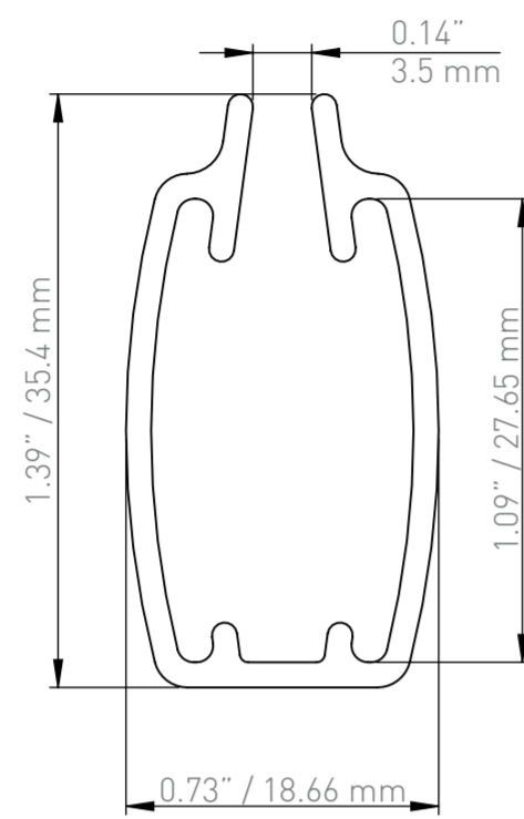
Neolux Bottomrail I 0-159-AL-0002X
