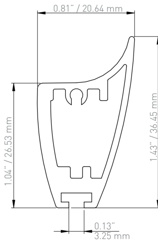
Neolux - Supreme Aluminum 0-159-AL-01XXX
