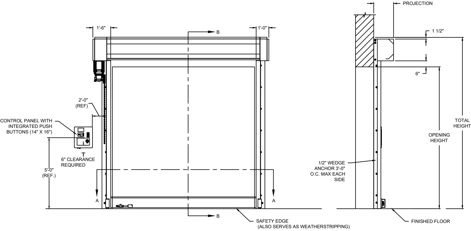
ELEVATION
