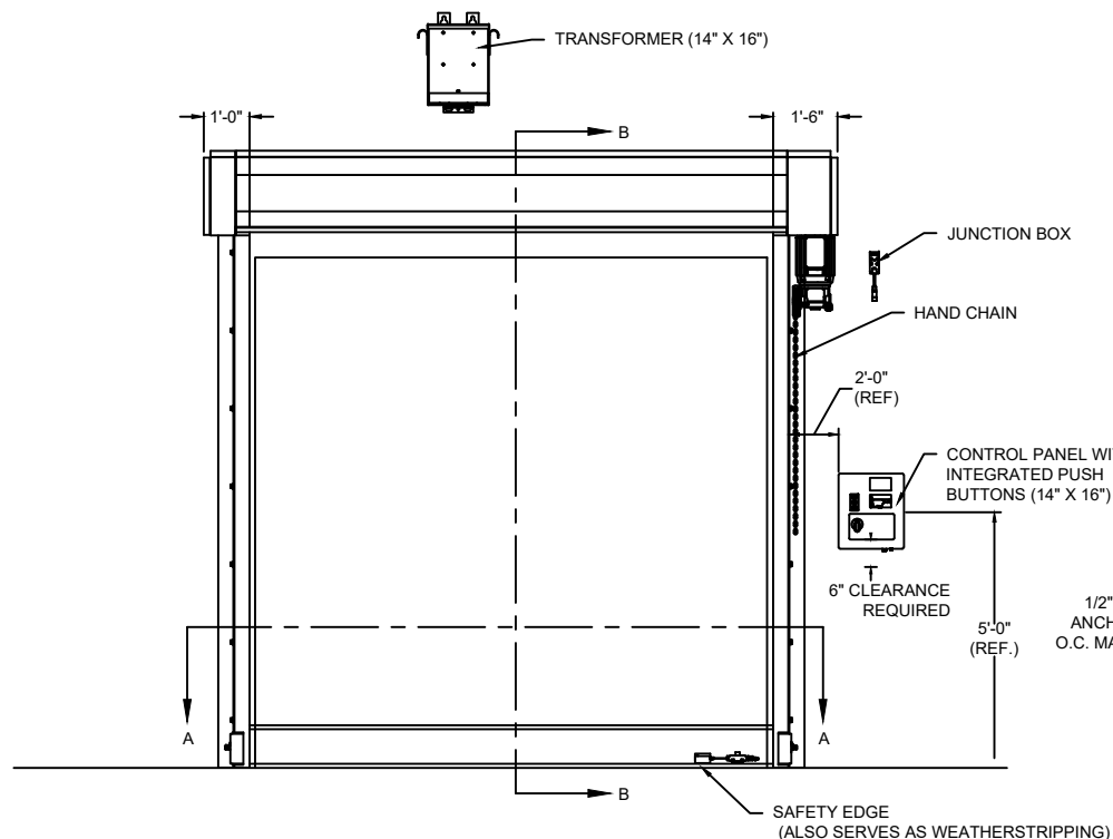
ELEVATION
