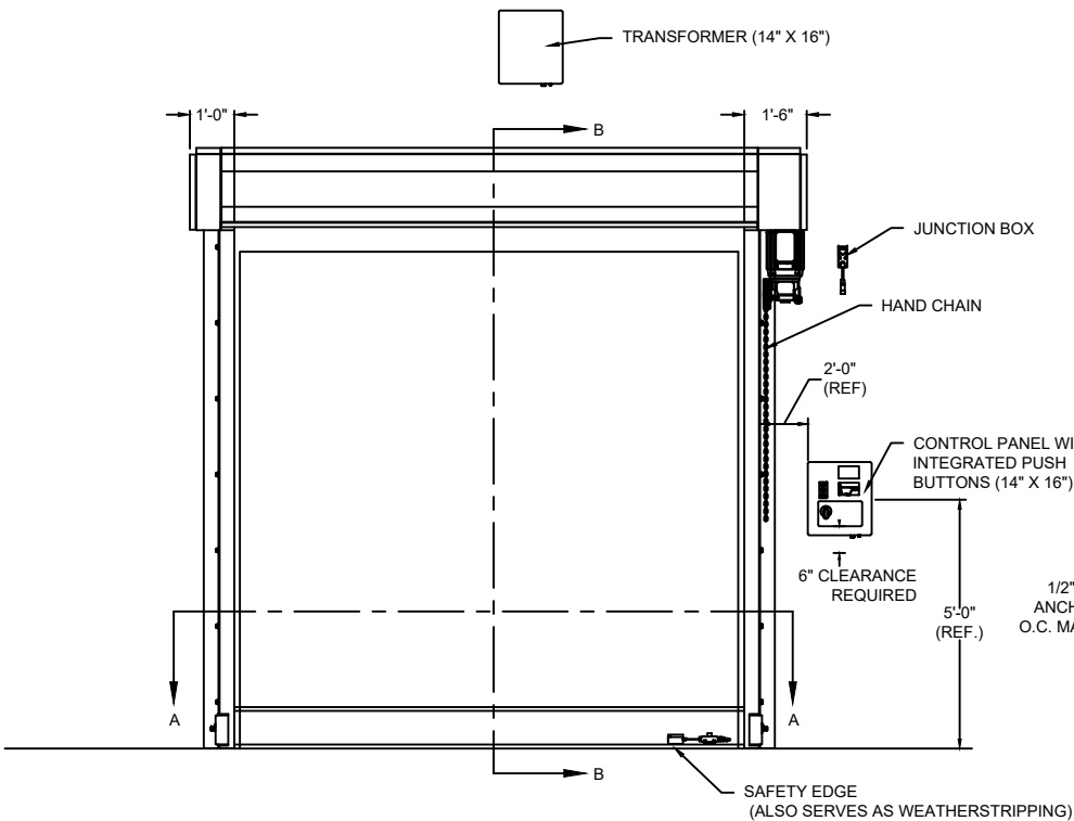
ELEVATION
