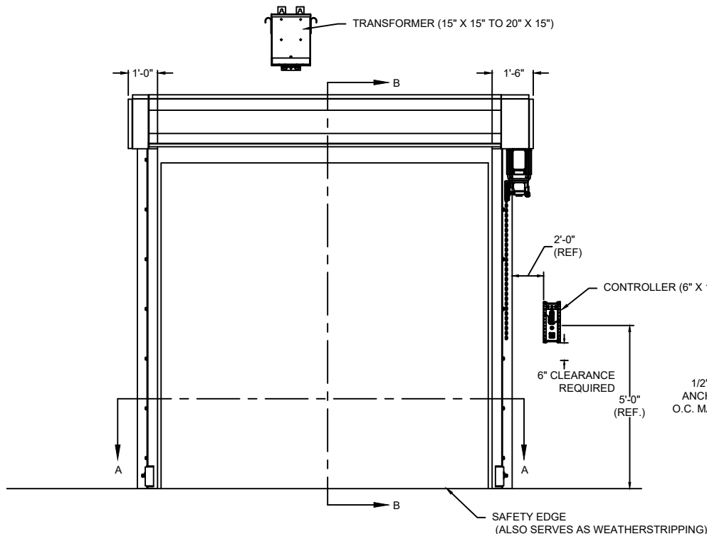
ELEVATION
