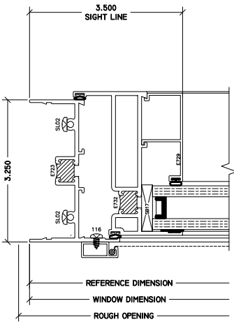
3 INSWING CSMT LJAMB 320 CASEMENT
