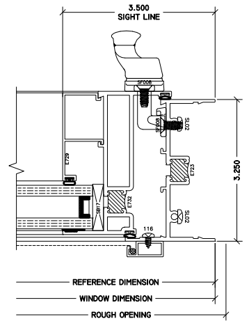
4 INSWING CSMT RJAMB 320 CASEMENT
