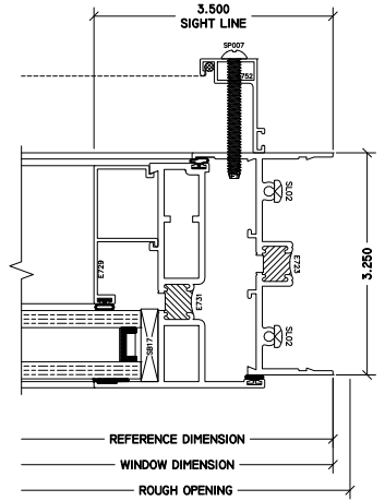
4 CASEMENT OUTSWING RJAMB 320 COL.
