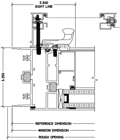
3 CASEMENT OUTSWING LJAMB 320 COL.
