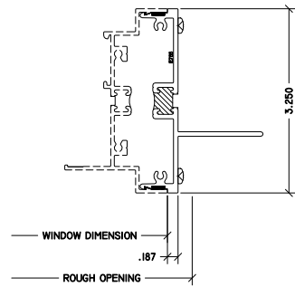
4 RIGHT JAMB NAIL FIN
