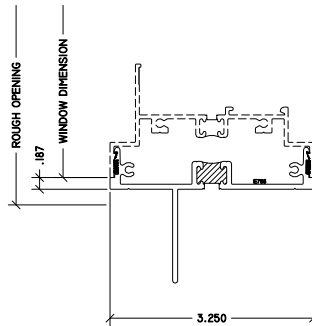
2 SILL NAIL FIN
