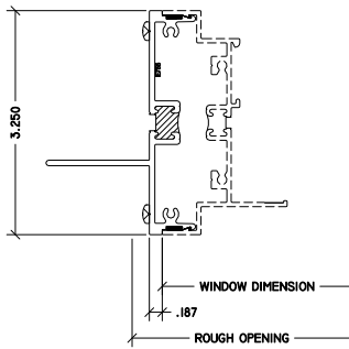
3 LEFT JAMB NAIL FIN
