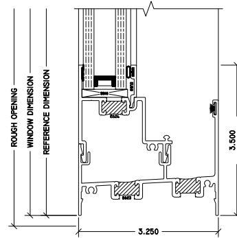
4 FX SILL 3210 HS
