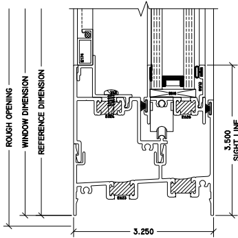
3 OP SILL 3210 HS
