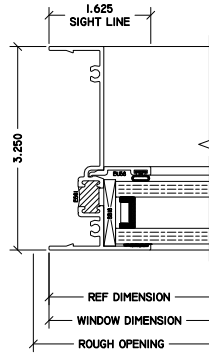
4 FX JAMB 3250 FXD
