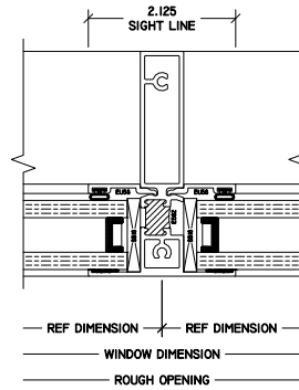
5 FX MUNTIN 3250 FXD
