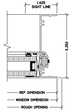
6 FX JAMB 3250 FXD
