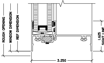
3 FX SILL 3250 FXD
