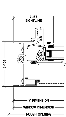
5 OP JAMB 210 SLIDER
