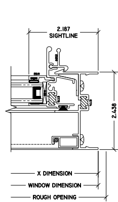
8 OP JAMB 210 SLIDER
