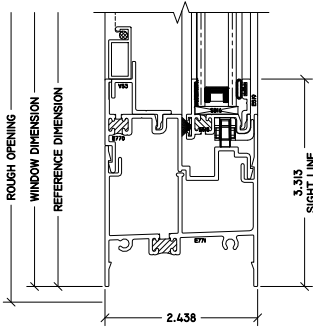
3 OP SILL 210 SLIDER
