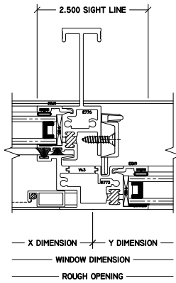
6 XO MTG. RAIL 210 SLIDER
