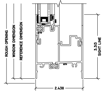
4 FX SILL 210 SLIDER
