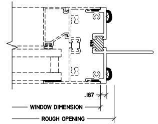
2 JAMB NAIL FIN
