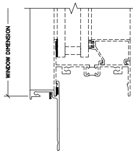
4 SILL STUCCO FIN
