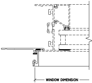
1 JAMB STUCCO FIN
