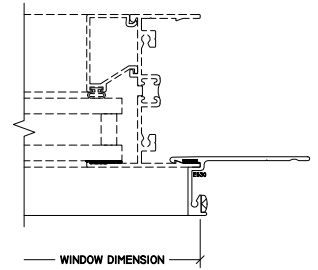
2 JAMB STUCCO FIN
