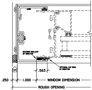
1 JAMB SUBFRAME
