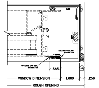
2 JAMB SUBFRAME
