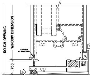
4 SILL SUBFRAME
