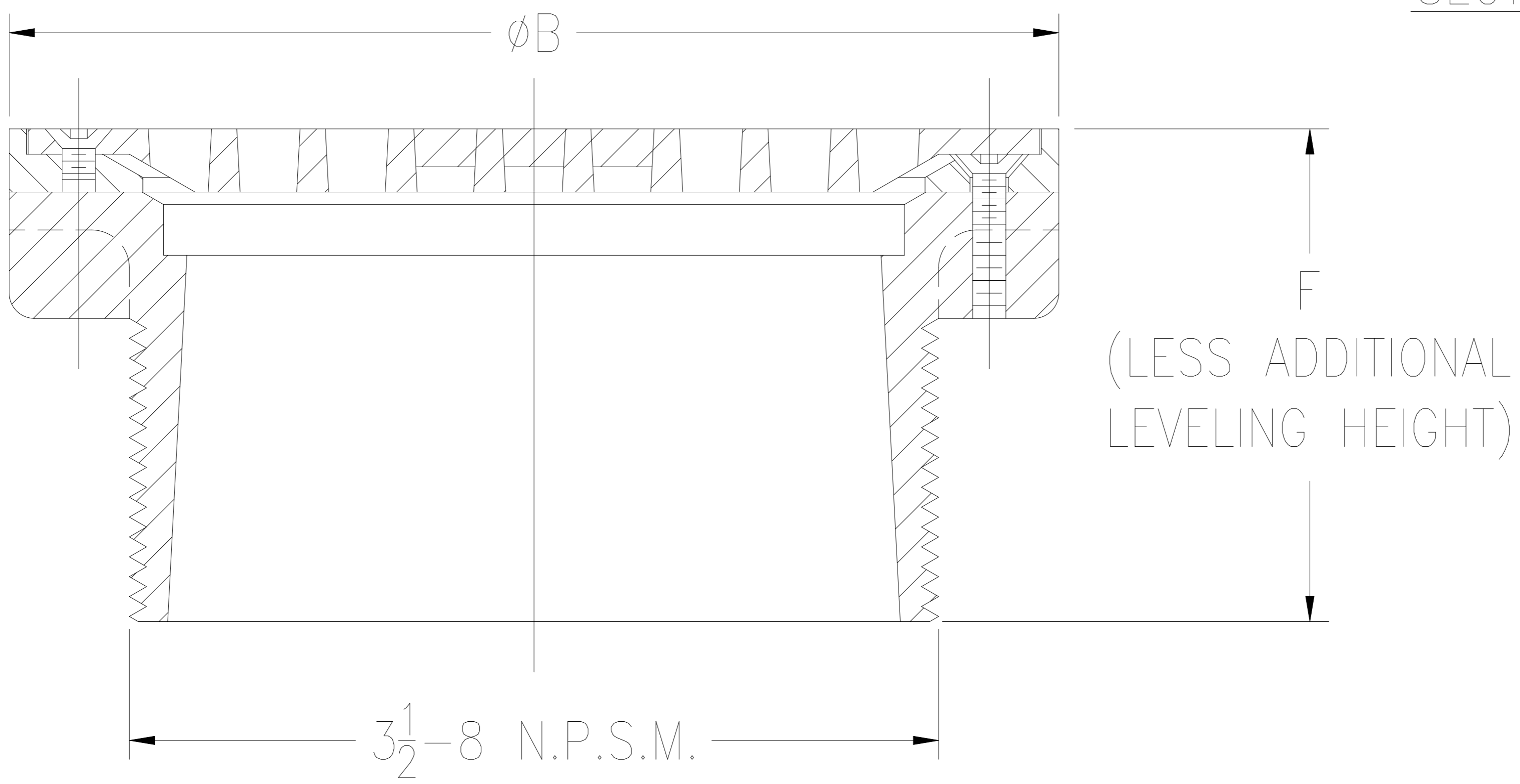
SECTION A-A
